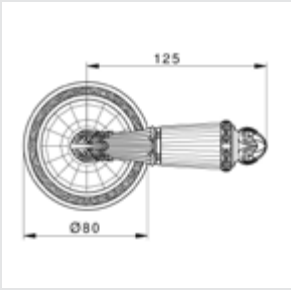
0R6220.000.** Door handle on roses
