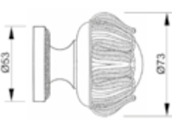
OC3016.000.** Door fixed knob
