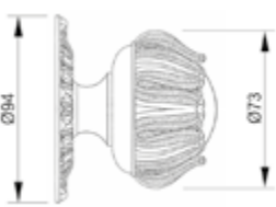
OC0651.652.** Door fixed knob
