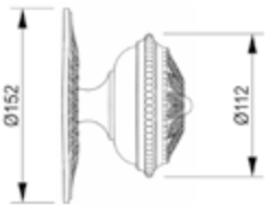
OC0860.861.** Door fixed knob
