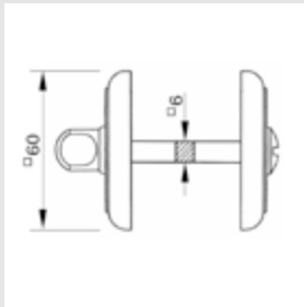
0WC064.6MM.** Privacy button
