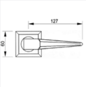
0R6454.000.** Door handle on roses
