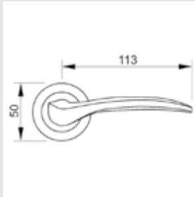
0R6751.000.** Door handle on roses
