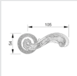
0R6516.000.** Door handle on roses
