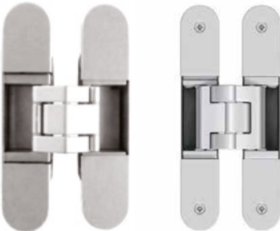
Cerniera a scomparsa porta a filo · Hidden hinge for flush door
