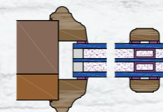
Vorsatzsprosse STIL Wiener Sprosse
