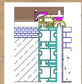
Bodeneinstandsprofil für thermische Trennung
